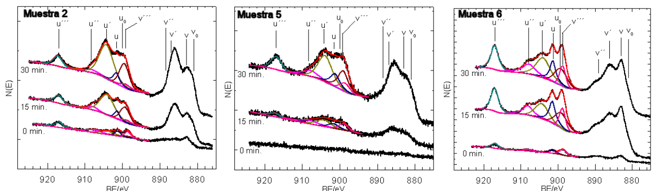
Figura 5. Espectros XPS de la componente Ce3d.
