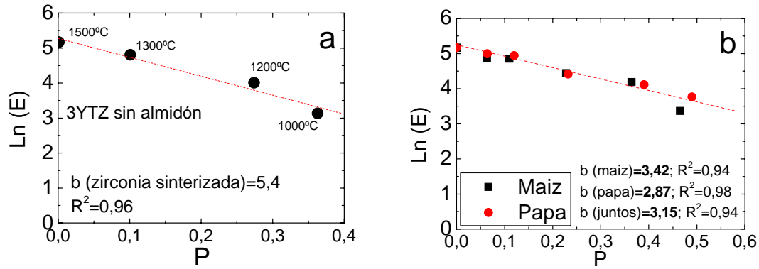
Figura 4: Variación de E con la porosidad de la zirconia porosa obtenida por diferentes métodos. a: sinterización parcial; b: con almidón de Maíz y Papa.
