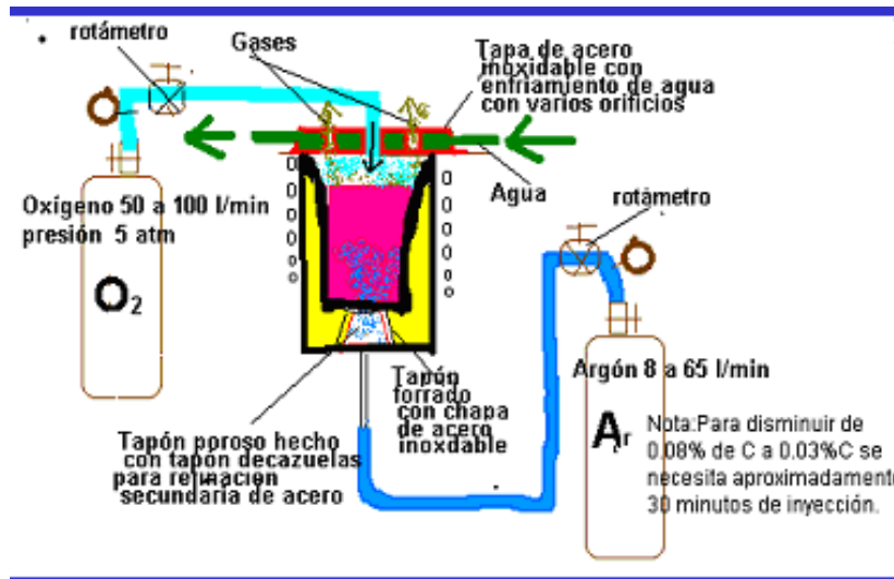
Fig 1.-Esquema de instalación del Horno de Inducción REACTOR.-con inyección de Argón por el fondo con un tapón poroso y Oxígeno por la parte superior del baño líquido con una lanza través de una tapa refrigerada con agua.
