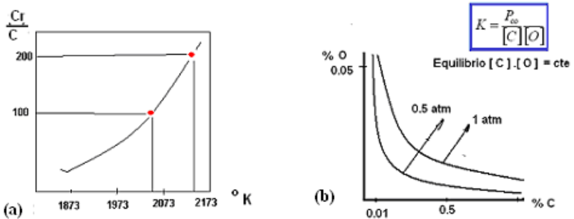
Fig 2. (a) Relación T^{\circ} K vs Cr / C . –(b) .-Equilibrio [C].[O]
