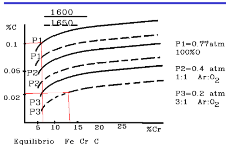
Fig 3.- Gráfico de equilibrio a partir de la ecuación de Hilty muestra la relación: [C] carbon en el metal; [Cr] en el metal; Temperatura del proceso y presión parcial de (CO) .
